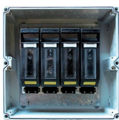
2x2-polig / 2x2-pole
