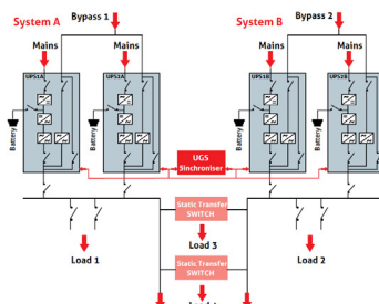
CONFIGURATION DYNAMIC DUAL BUS Solution qui assure la redondance jusqu'à la distribution de l'alimentation aux charges et un meilleur fonctionnement des STS. + Discrimination des pannes en aval
