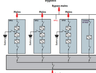
JUSQU'À 8 ASI EN CONFIGURATION PARALLÈLE AVEC BYPASS COMMUN + Sélectivité des défauts en aval en mode bypass
