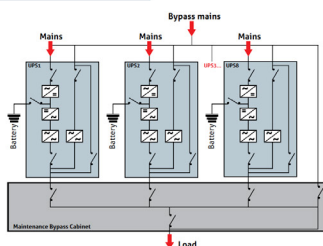
JUSQU'À 8 ASI EN CONFIGURATION PARALLÈLE AVEC BYPASS DISTRIBUÉ + Flexibilité et modularité sans point de défaillance unique.
