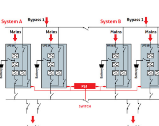
CONFIGURATION DUAL BUS SYSTEM Solution qui assure la redondance de l'alimentation même pendant la maintenance. + Haute disponibilité et redondance
