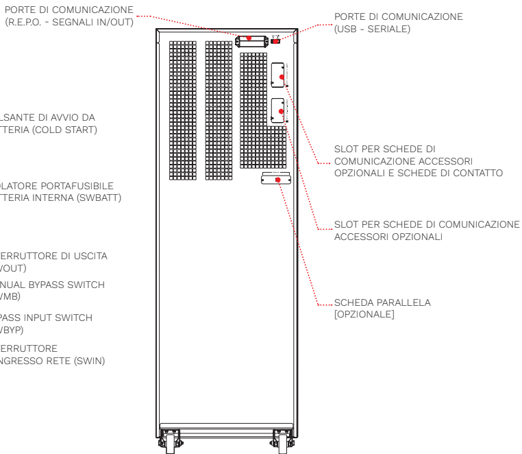
XTEND 60 kVA (retro)
